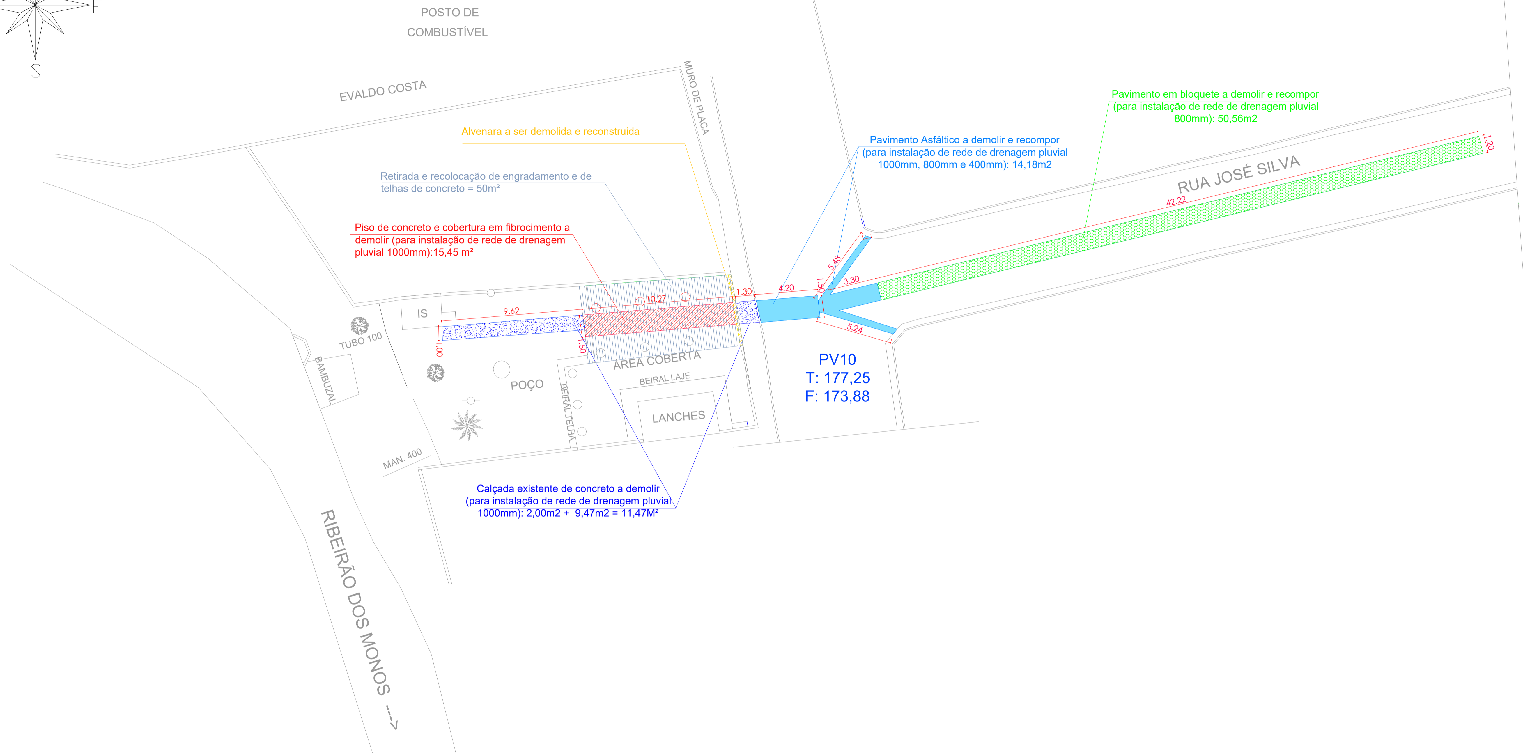
PLANTA BAIXA DE DEMOLIÇÕES E CONSTRUÇÕES (Rua José Silva - parte 1) ESCALA 1/150
