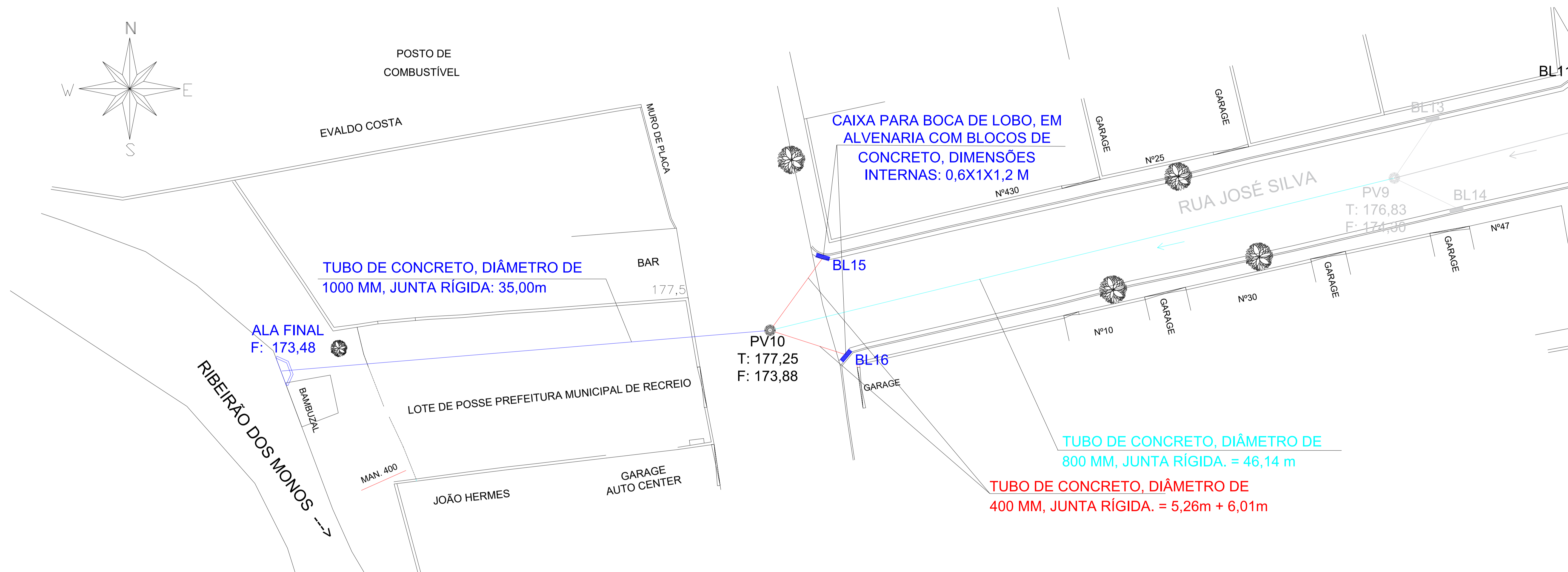
PLANTA BAIXA DE DRENAGEM PLUVIAL (Rua José Silva e Área de Servidão) ESCALA 1/150
