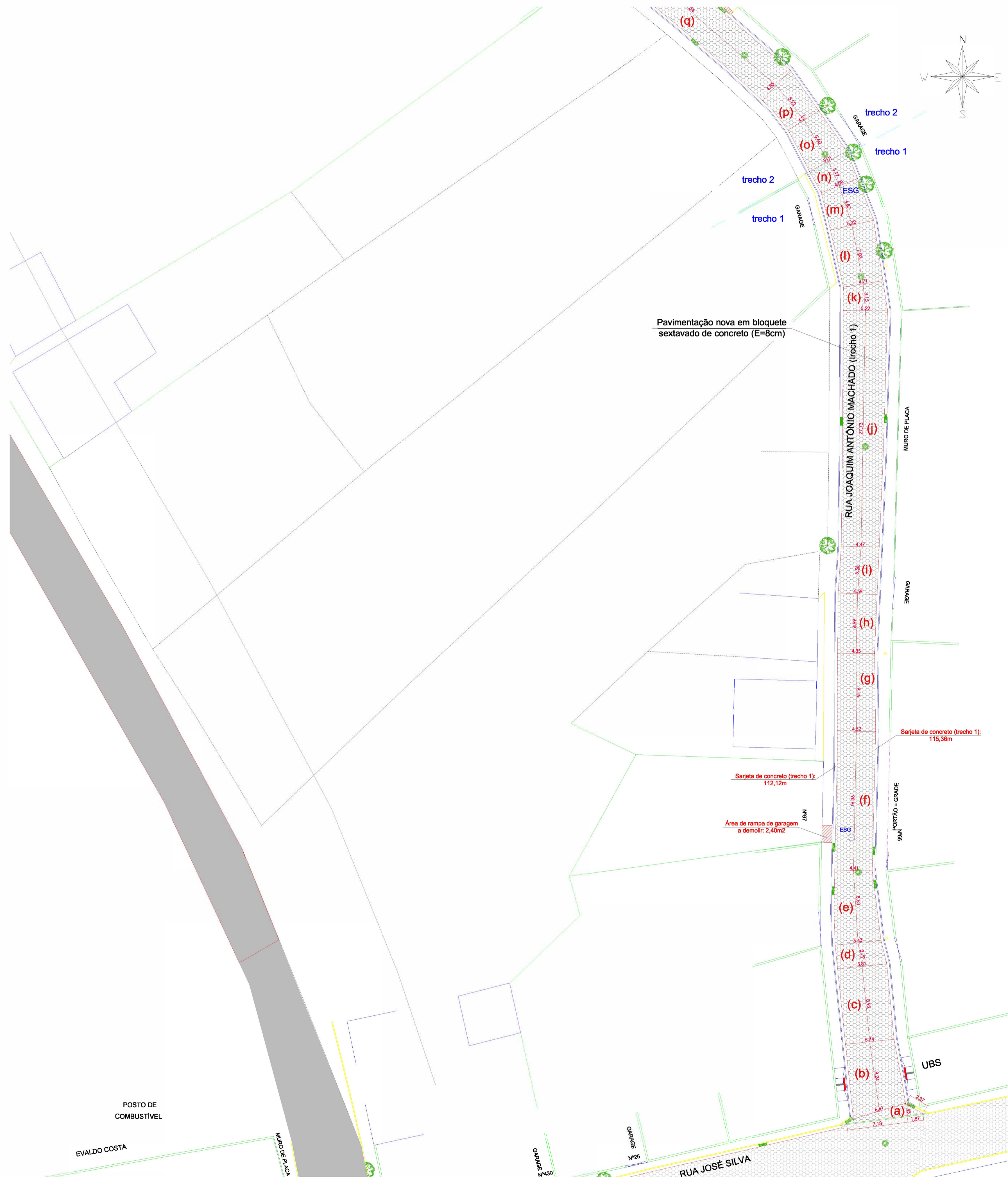
PLANTA BAIXA DE PAVIMENTAÇÃO (Rua Joaquim Antônio Machado - parte 2) ESCALA 1/250
