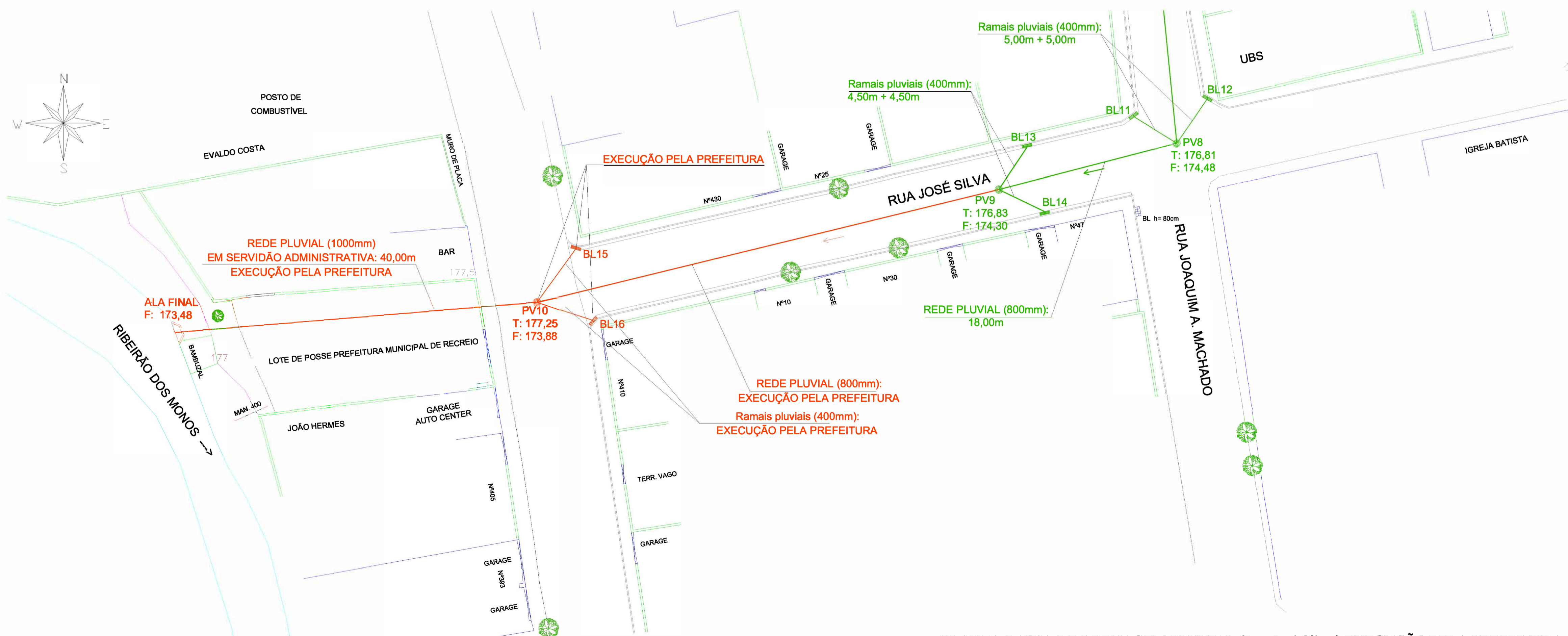
PLANTA BAIXA DE DRENAGEM PLUVIAL (Rua José Silva) EXECUÇÃO PELA PREFEITURA ESCALA 1/250
