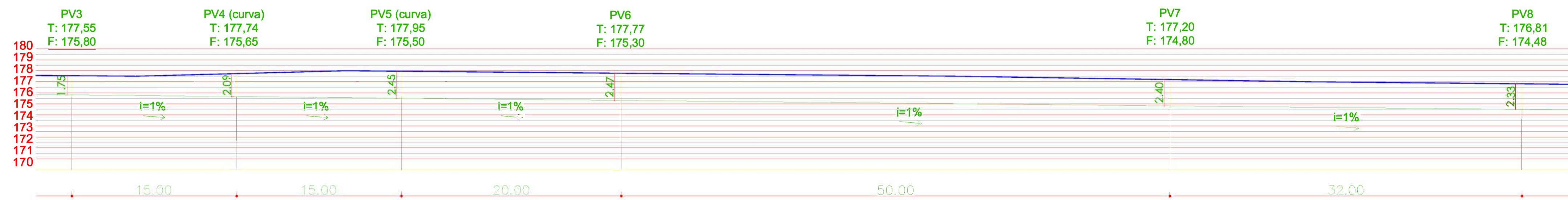
CORTE LONGITUDINAL DE DRENAGEM (Rua Joaquim Antônio Machado - parte 2) ESCALA 1/250
