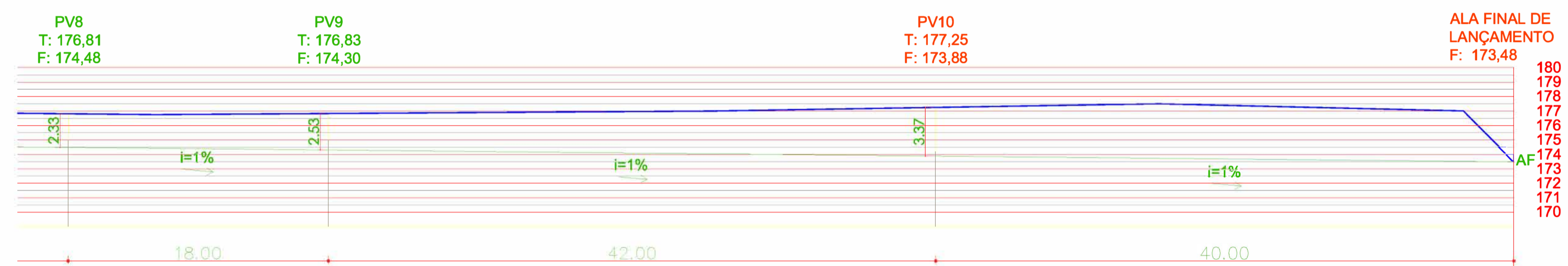
CORTE LONGITUDINAL DE DRENAGEM (Rua Joaquim Antônio Machado - parte 3) ESCALA 1/250
